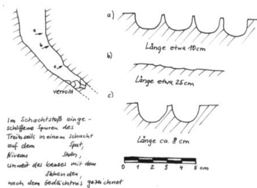
Abbildung 20: Schleifspuren des Treibeseils im Hangenden eines Schachts
