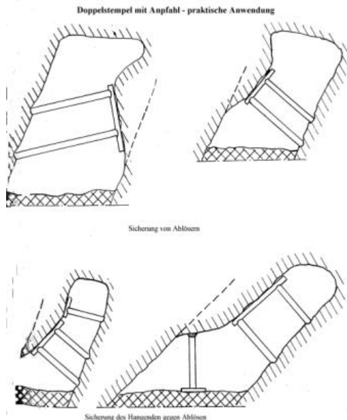
Abbildung 93: Einsatzbeispiele des Doppelstempels mit Anpfahl nach: [32]
