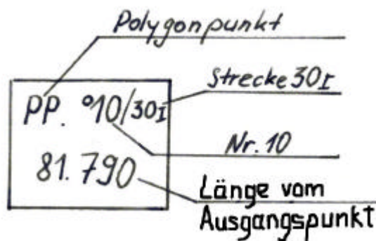
Abbildung 37: Polygonpunkttafel
