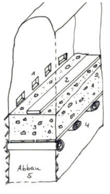
Abbildung 124: Hinweise auf Hohlräume unter Strecken
