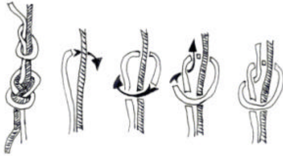
Abbildung 135: Zusätzlicher Sicherungsknoten
