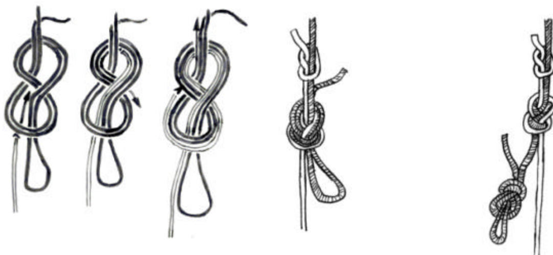
Abbildung 167: Umsteigestelle im frei hängenden Seil mit speziellem Achterknoten
