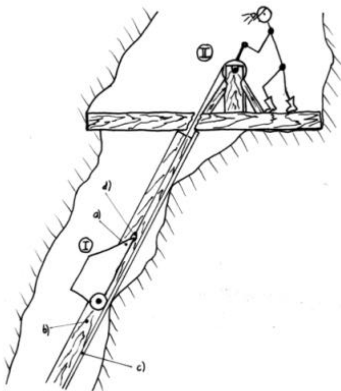
Abbildung 77: Einbau eines Haspels im Schacht
