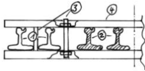
Abbildung 75: "Wechsel" für teilweise aufgetrennte Verwahrungen
