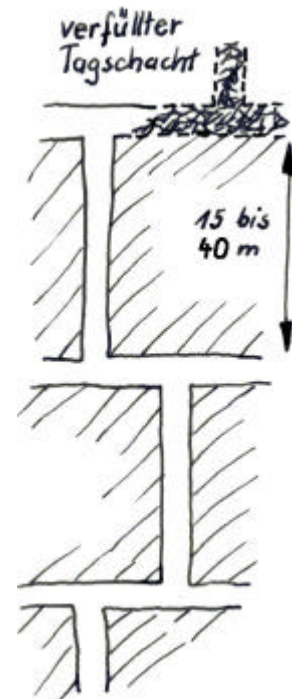
Abbildung 13: Abgesetzte Schächte
