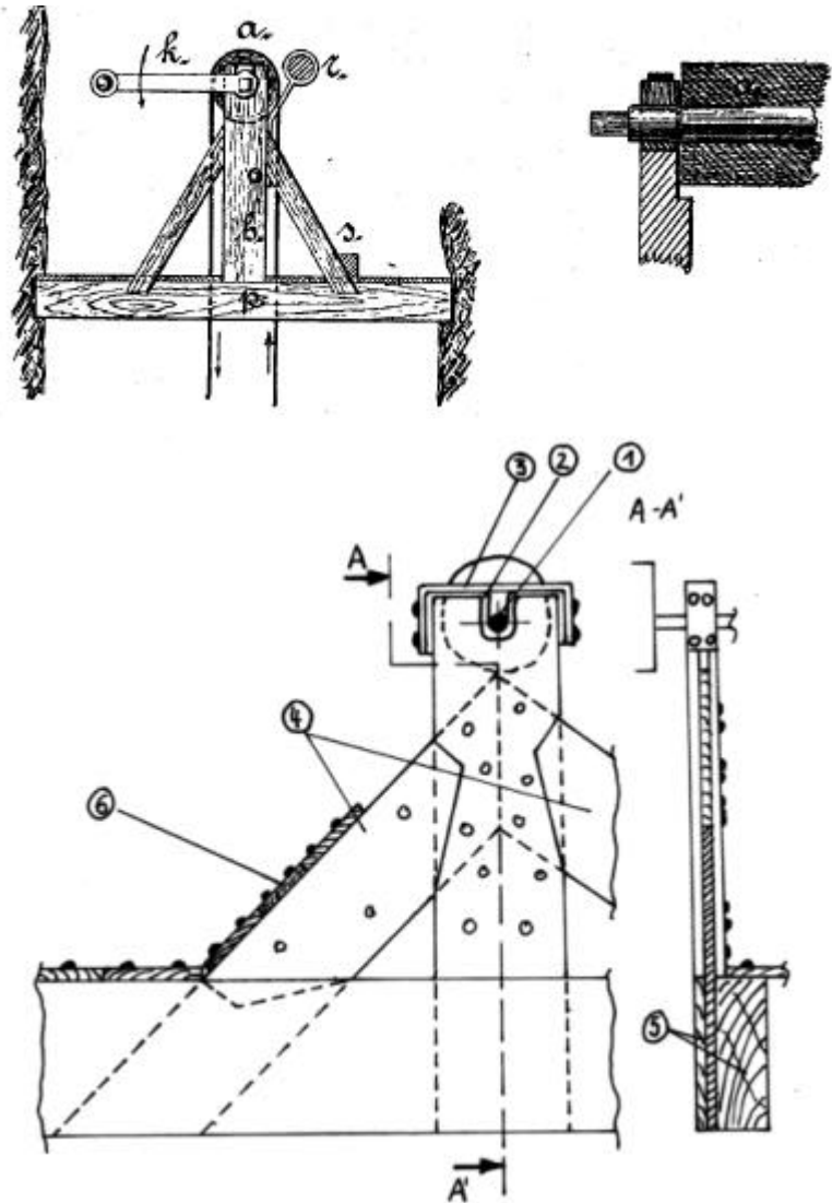
Abbildung 76: Konstruktionen für Haspel
