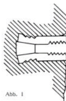
Abbildung 155: Sauber gesetzter Spit Nach Weber, D. in [5]
