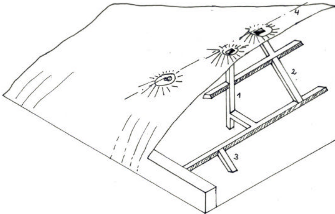
Abbildung 14: Schächte: Begriffe
