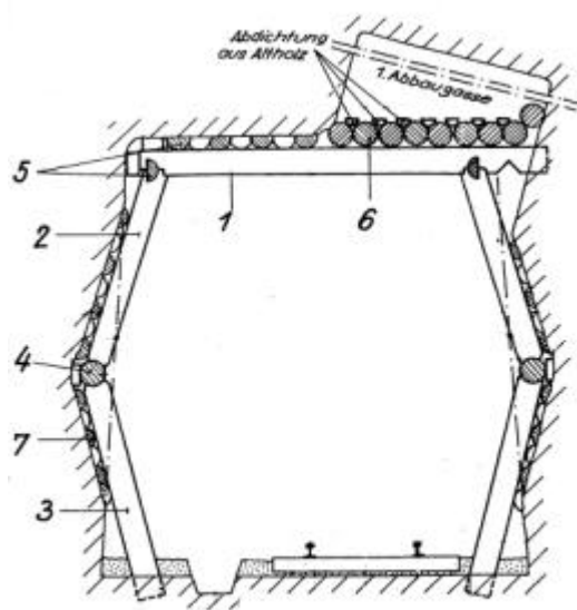
Abbildung 95: Offener Polygonausbau
