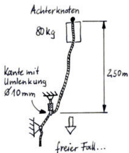
Abbildung 131: Aufbau eines Normsturzversuchs ähnlich Stark verändert nach [5], Ausg. 9 UIAA
