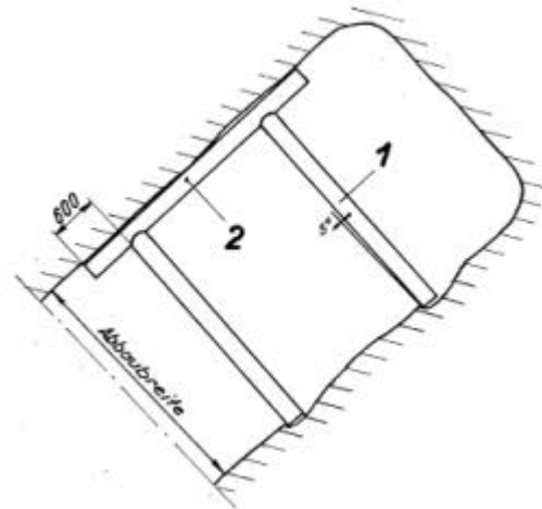
Abbildung 92: Doppelstempel mit Anpfahl, Prinzip
