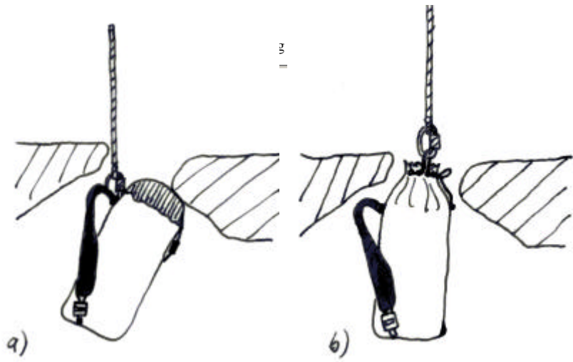
Abbildung 54: Lage der Rucksackaufhängung
