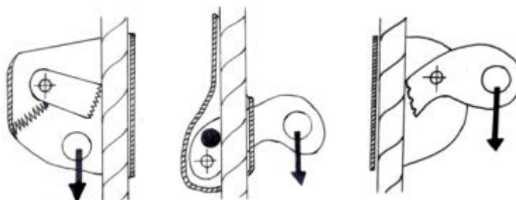
Abbildung 141: Verschiedene Funktionsprinzipien von Seilklemmen
