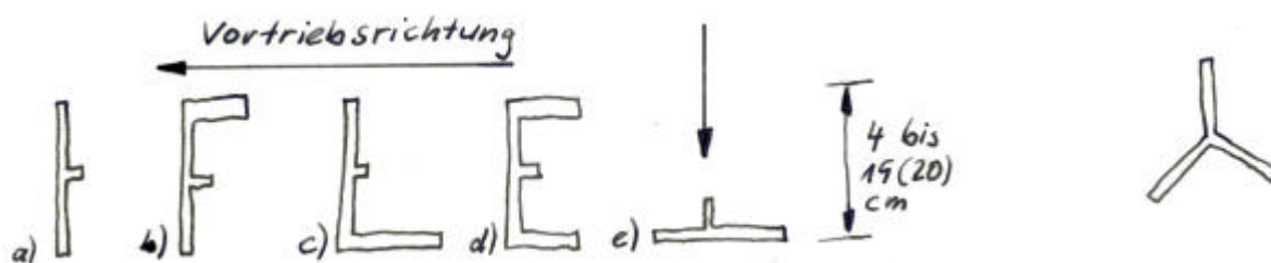
Abbildung 32: Freiburger Gedinge
