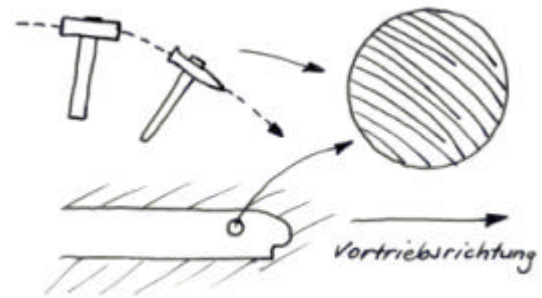
Abbildung 16: Arbeit mit Schlegel und Eisen
