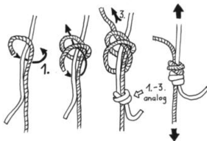
Abbildung 139: Legen eines doppelten Spierenstichs
