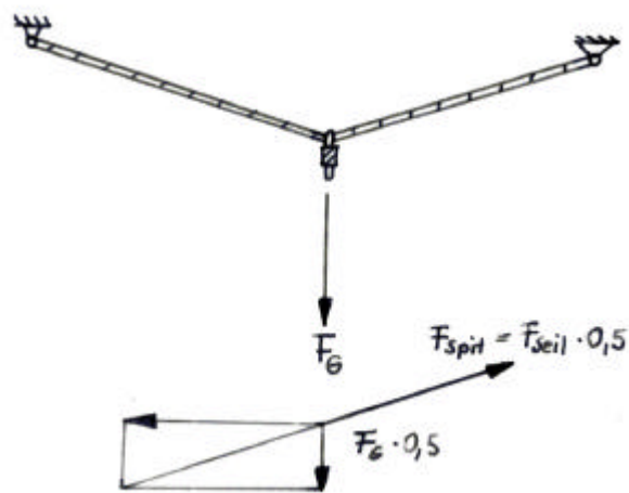
Abbildung 174: Kräfteverhältnisse am Quergang
