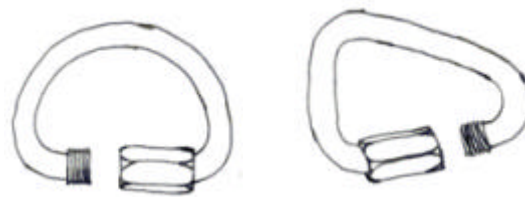
Abbildung 148: Formen für Zentral-Schraubglieder Links) Günstige D-Form; Rechts) ungünstigere Delta-Form
