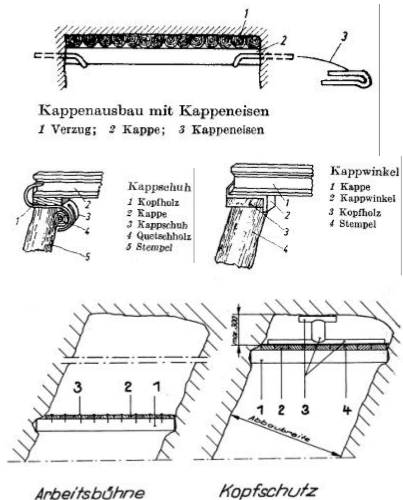
Abbildung 94: Ausbau mit Kappen
