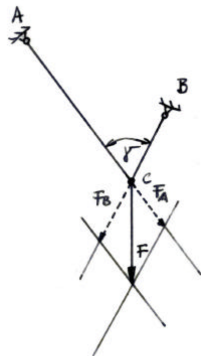
Abbildung 158: Kräfteverhältnisse an einer Zwei-Punkt-SeilAufhängung
