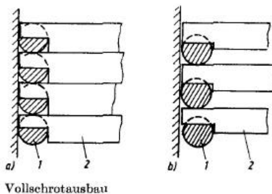
Abbildung 110: Vollschrötausbau aus [30]
