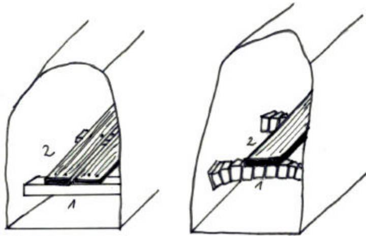
Abbildung 45: Tragewerk
