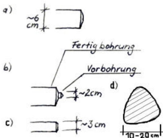
Abbildung 18: Bohrlochformen
