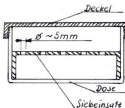
Abbildung 52: spezielle Karbiddose
