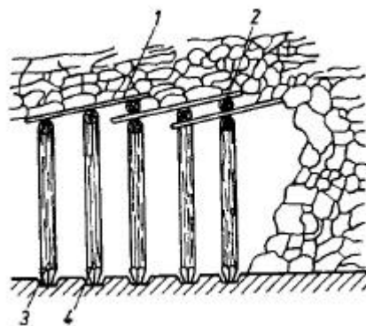
Abbildung 89: Nachgiebig gestalteter Stempel am Beispiel einer Getriebezimmerung
