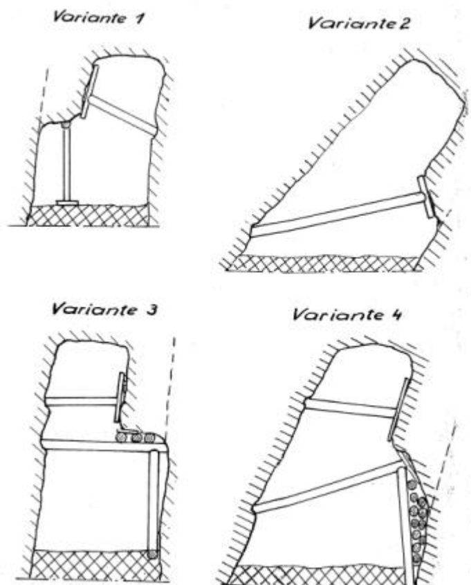
Abbildung 91: Einsatzbeispiele des Stempels mit Anpfahl nach: [32]
